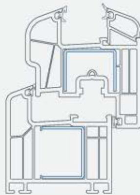
Arcade półzlicowane
